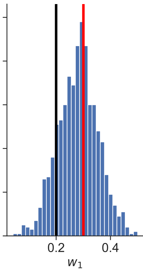
Posterior distributions Dataset 28
