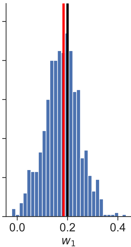
Posterior distributions Dataset 22
