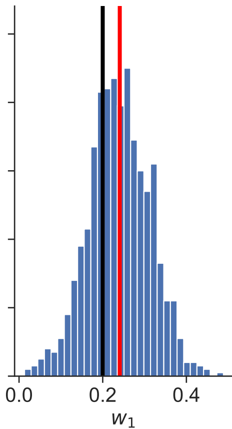
Posterior distributions Dataset 21
